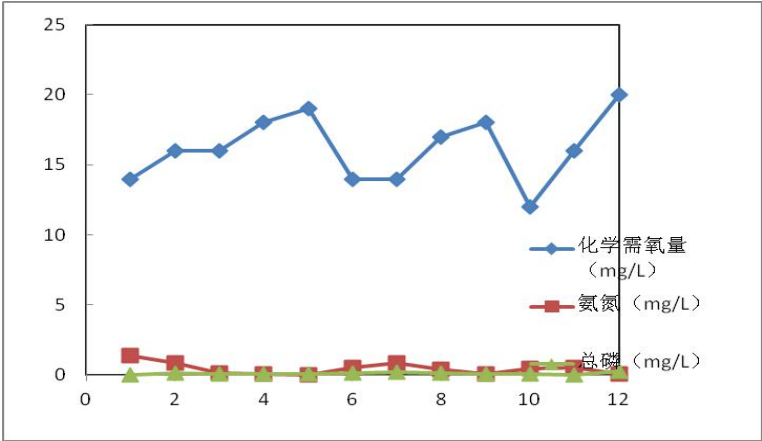
图 1-3 2020 年白马河捷庄断面化学需氧量、氨氮、总磷比较
