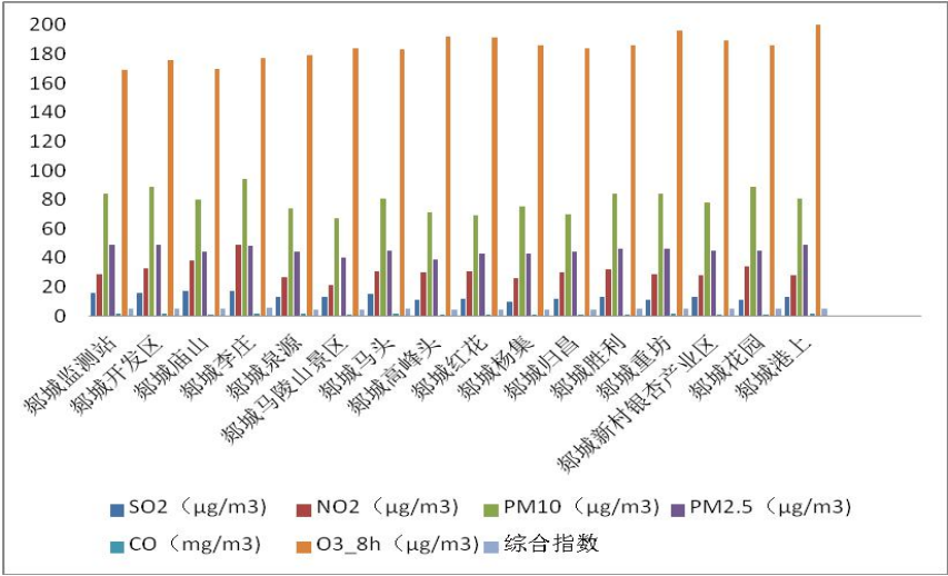
图 3-1 各站点污染物项目浓度年均值对比图
