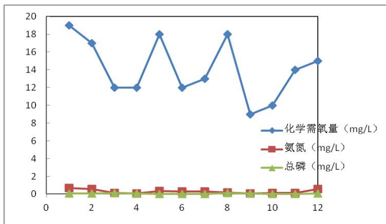
图 1-1 2020 年沂河鲁苏省界断面化学需氧量、氨氮、总磷比较
