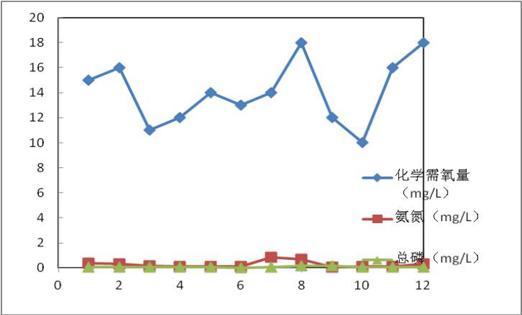
图 1-2 2020 年沭河小李庄桥断面化学需氧量、氨氮、总磷比较
